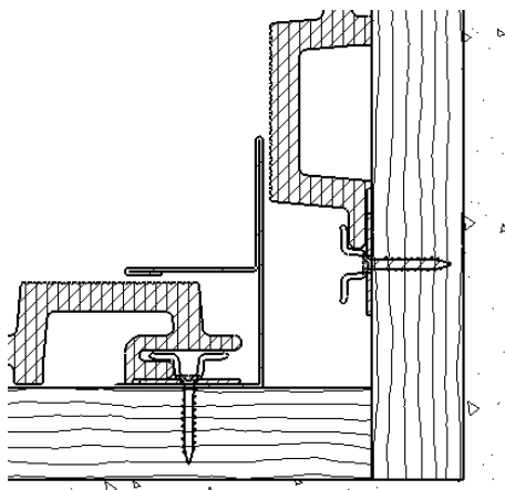
ANGLE RENTRANT
