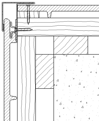
ANGLE SORTANT
