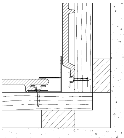
ANGLE RENTRANT
